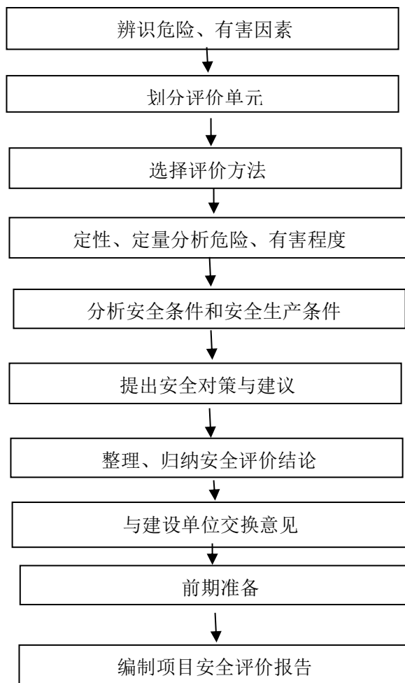
图 1-1 安全验收评价程序框图
